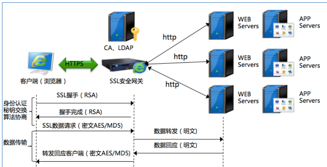
SSL 安全网关方案图示
